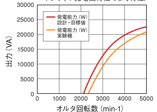
ハイブリッド発電機特性 (冷時特性)
